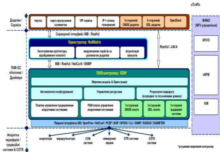
Рисунок 2 – Загальна розширена структура мереж SDN
