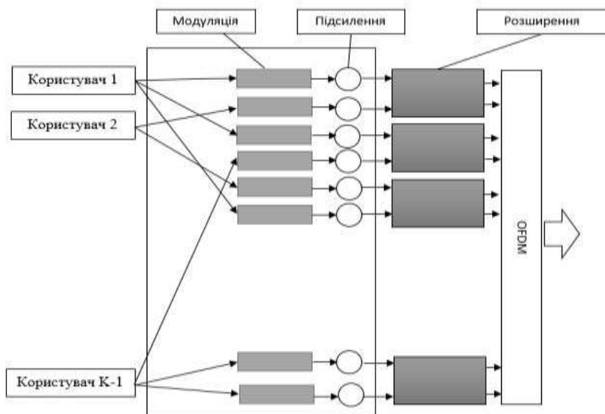
Рисунок 1 - Архітектура системи для оптимізації
