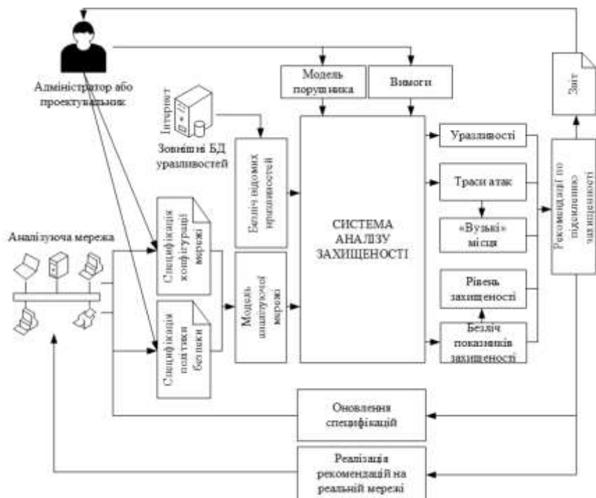
Рисунок 1 – Представлення системи аналізу захищеності
