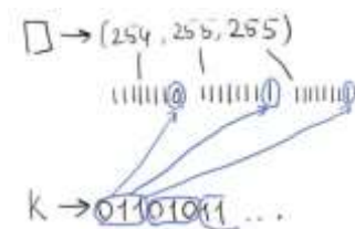
Рисунок 3- Заміна молодшого біта каналу кольору на біт тексту.
