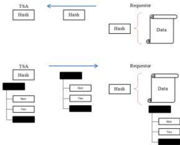
Рисунок 2 - Порядок реєстрації даних
