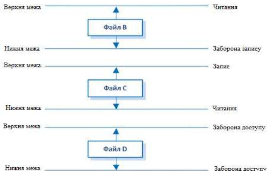
Рисунок 2 – Модель інформаційної безпеки Кларка-Уїлсона.
