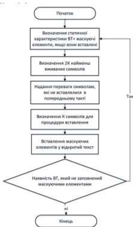
Рисунок 1 - Загальна схема алгоритму вставлення маскуючих елементів
