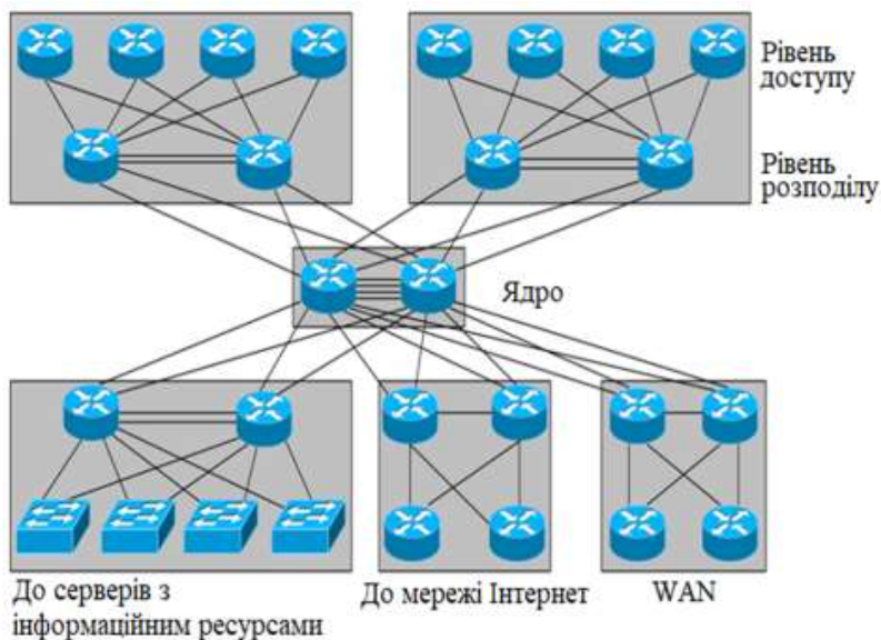
Рисунок 1 – Трирівнева ієрархічна модель побудови мережі
