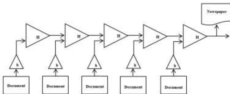
Рисунок 1- Лінійна схема об'єднаних хешів
