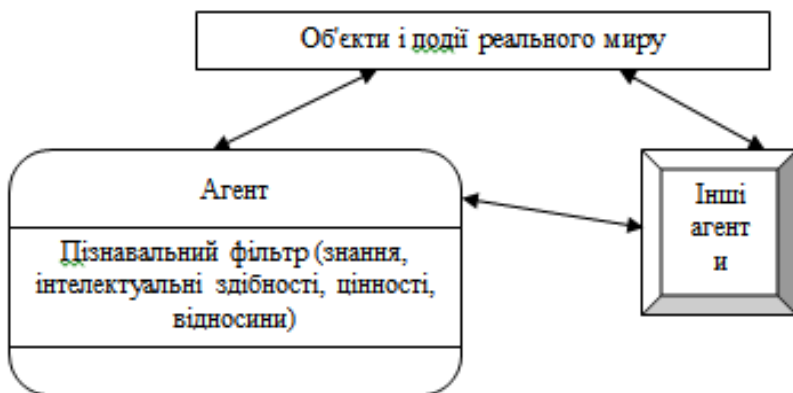
Рисунок 1 – Інтелектуальний агент
